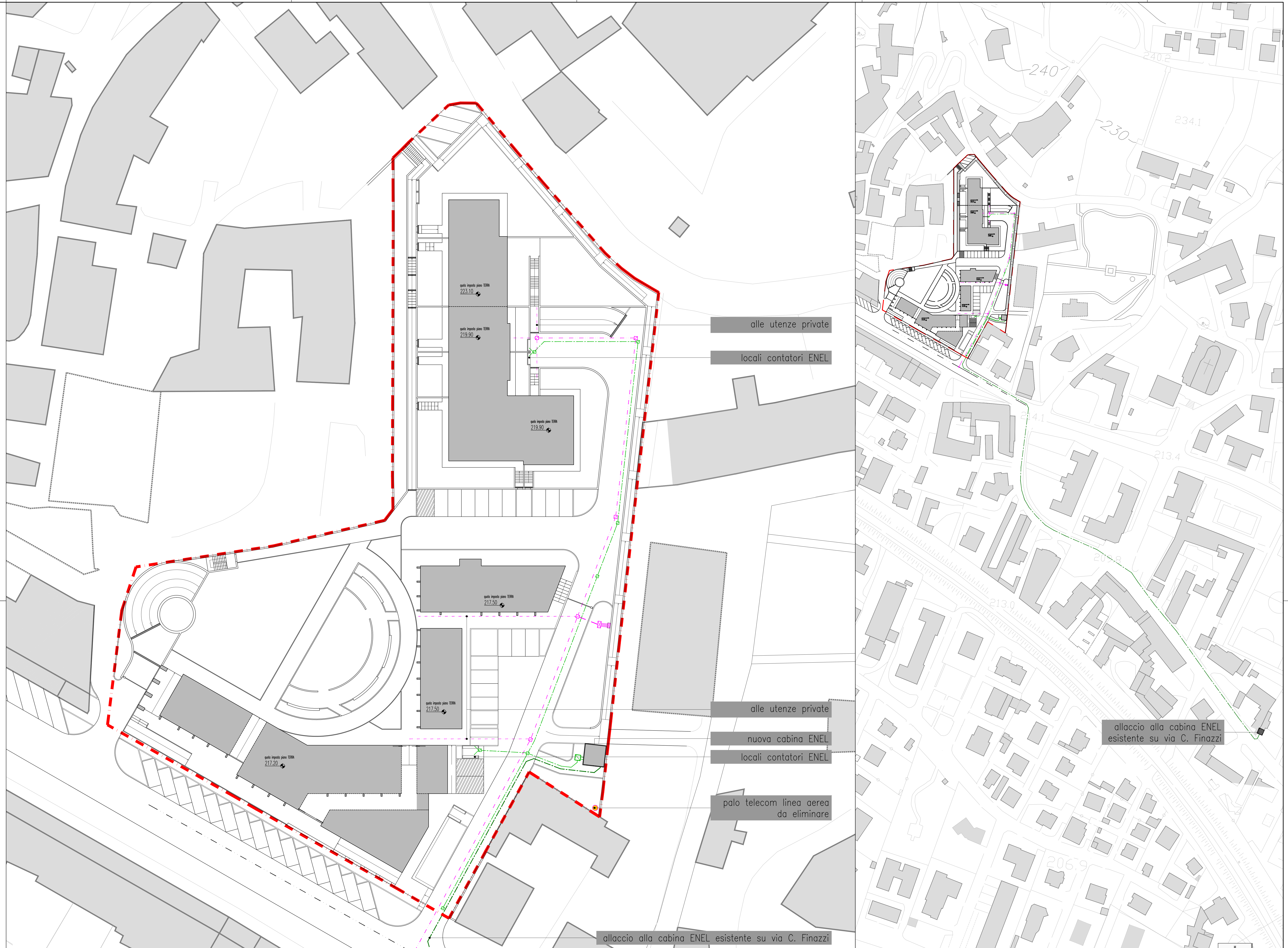
PLANIMETRIA GENERALE _ RETE DISTRIBUZIONE ENERGIA ELETTRICA e TELECOMUNICAZIONI
